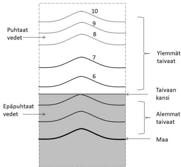
Kuva 5. Taivaankannen luominen puhtaiden ja saastuneiden taivaiden väliin.
