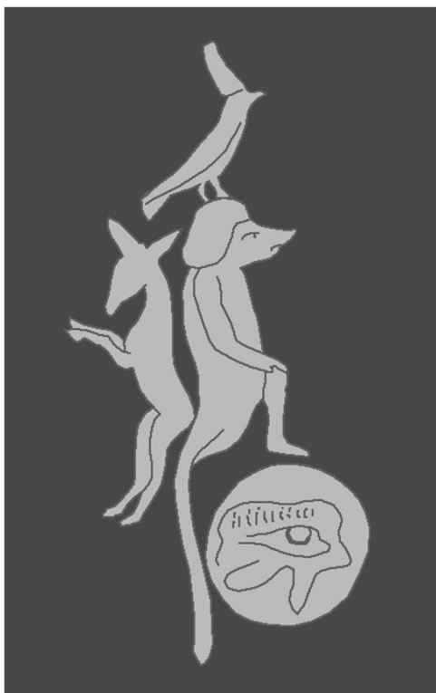
Kuva 28. Aasi ja Peto Denderan kartastossa.
