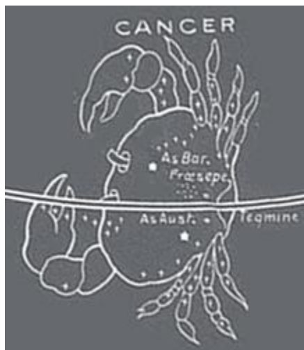
Kuva 46. Klassinen Krapu (Bullinger).
