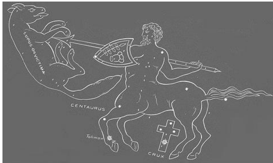
Kuva 8. Klassiset Kentaurin (Centaurus) ja Suden/Uhrin (Lupus/Victima) kuviot Bullingerin piirroksen mukaan.
