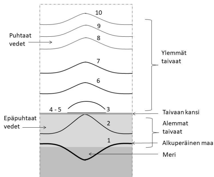
Kuva 37. Sielujen maailma ensimmäisen ylösnousemuksen jälkeen. Paratiisi (3) on nostettu taivaankannen yläpuolelle. Tuonela (2) on sen jälkeen ylin taso sielujen maailmassa ja Kristus on asettanut merkkiviirinsä sen huipulle. Viimeinen pelastusoperaatio kohdistetaan kaikkialle sielujen alamaailmaan eli Kuolemaan (1) ja Tuonelaan.
