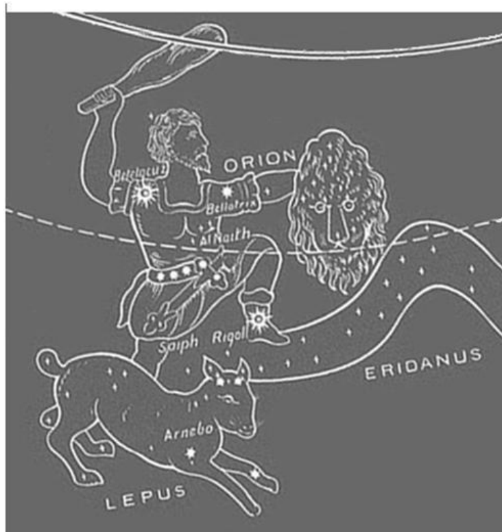
Kuva 40. Orionin klassinen kuvio (Bullinger).
