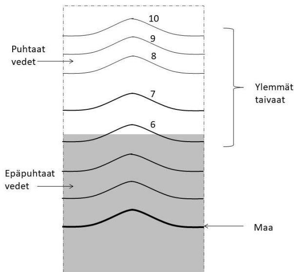
Kuva 4. Henkien/enkelien maailman (6. taivas) puhdistaminen.
