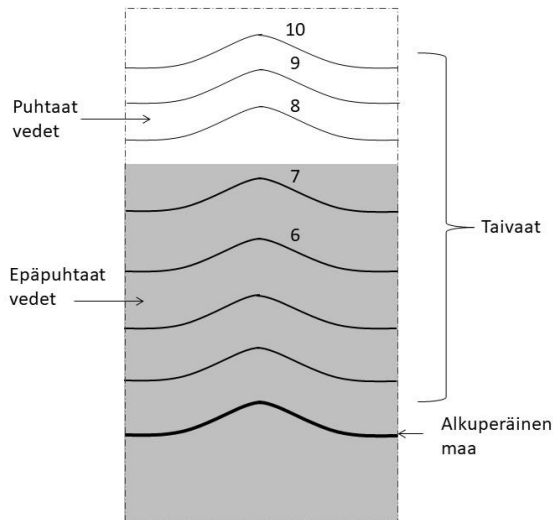
Kuva 3. Saastaisten vesien nouseminen alkuperäisen näkymättömän maan ja näkymättömien taivaiden yläpuolelle. Numerot viittaavat taivaiden järjestyslukuun. 20
