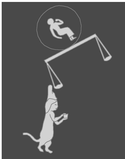
Kuva 10. Uhri (Victima) ja Vaaka (Libra) Denderan tähtikartastossa.
