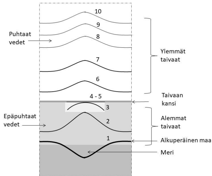
Kuva 21. Sielujen maailma taivaankannen alapuolella ja ylemmät puhdistetut taivaat taivaankannen yläpuolella. 1. Kuolema (alkuperäinen näkymätön maa ja meri), 2. Tuonela (alkuperäinen sielujen taivas), ja 3. Paratiisi.
