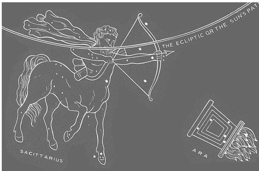
Kuva 18. Jousimiehen (Sagittarius) ja Alttarin (Ara) kuviot Bullingerin mukaan.
