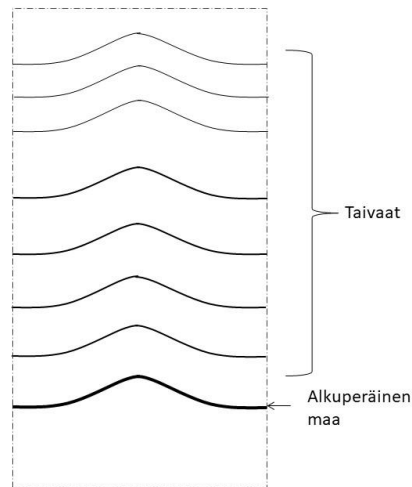
Kuva 2. Alussa Jumala loi taivaat ja maan eli näkymättömän luomakunnan. Alimpana oli alkuperäinen näkymätön maa. Sen yläpuolella oli monta taivasta. Kuva on periaatteellinen, koska kaikkia näkymättömän luomakunnan ulottuvuuksia ei voida siinä esittää. 19
