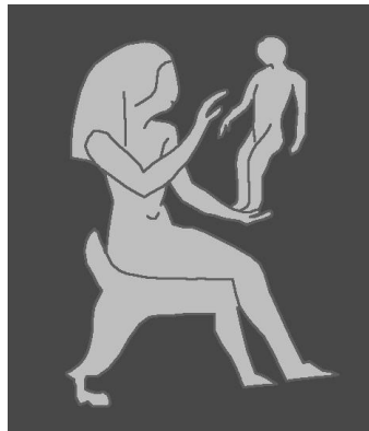
Kuva 7. Coma Denderan tähtikartastossa.
