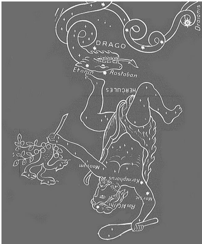
Kuva 15. Lohikäärme (Draco) ja Herkules Bullingerin mukaan.
