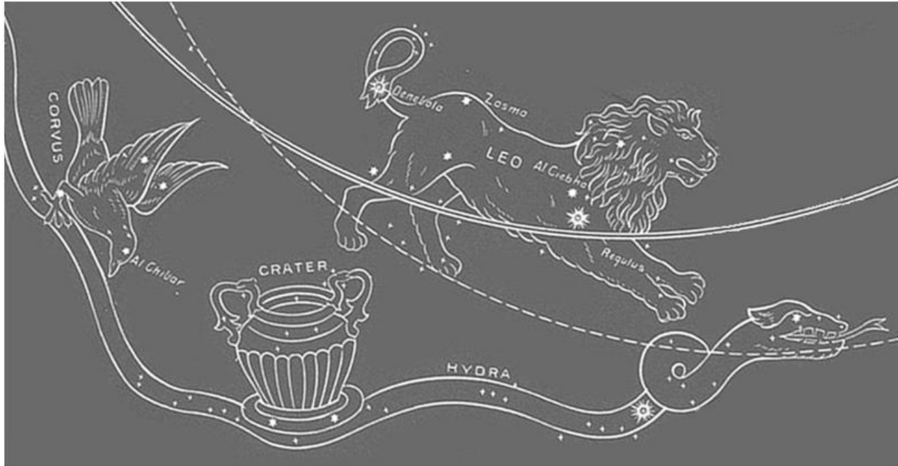
Kuva 49. Leijona (Leo), Vesikäärme (Hydra), Malja (Crater) ja Korppi (Corvus) klassisesti esitettynä (Bullinger).
